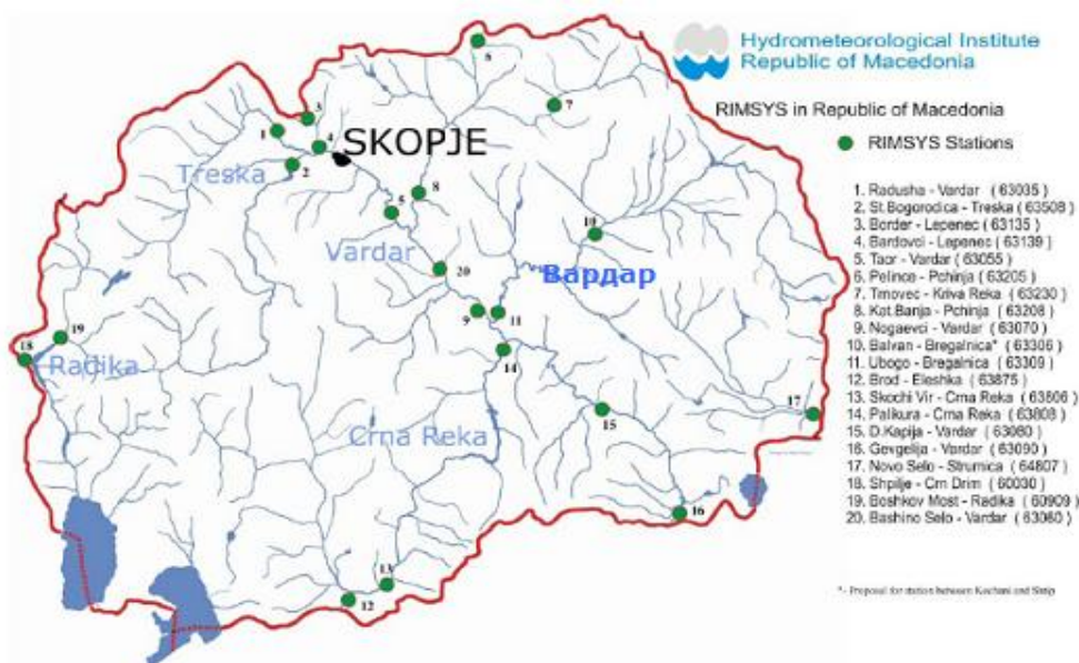
Слика 16: RIMSIS станици за мониторинг на водотеци
